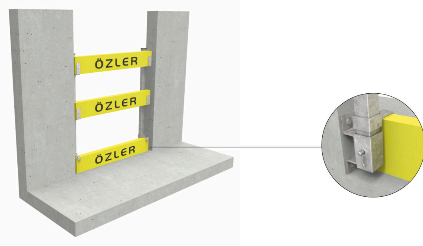
SAFETYBOARD Açı Ayarlı Taban Plakası Montajı SAFETYBOARD Articulated/Hinged Panel Assembly
